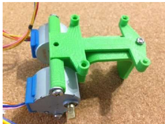
Figura 7. Vista de montaje de soportes.
