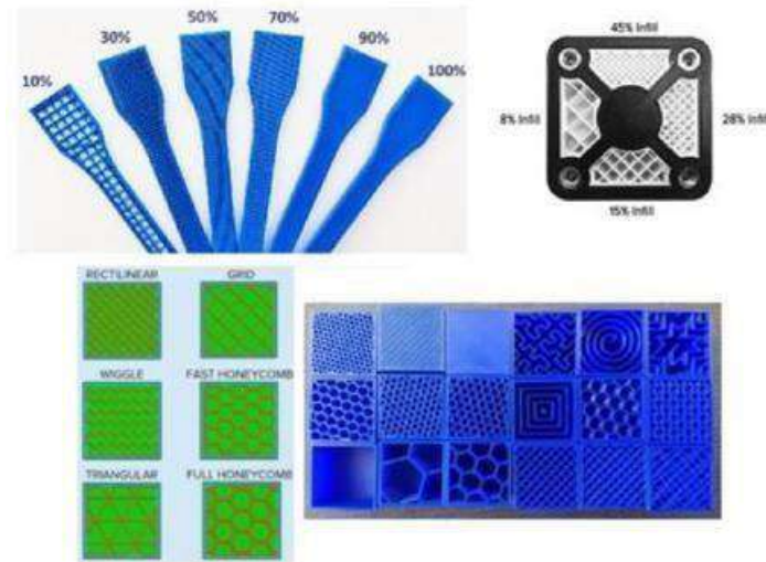
Figura 7. Rellenos en impresión 3D.
