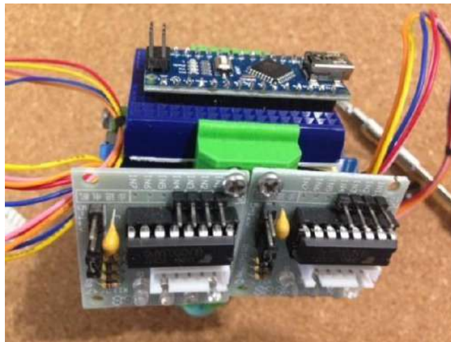
Figura 16. Vista general.
