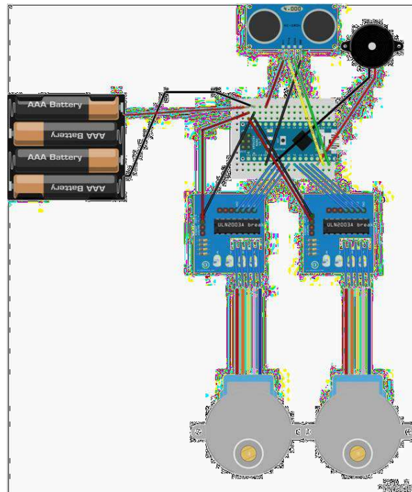
Figura 16. Conexión de los motores al arduino.
