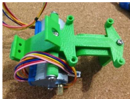
Figura 9. Vista del montaje de los motores
