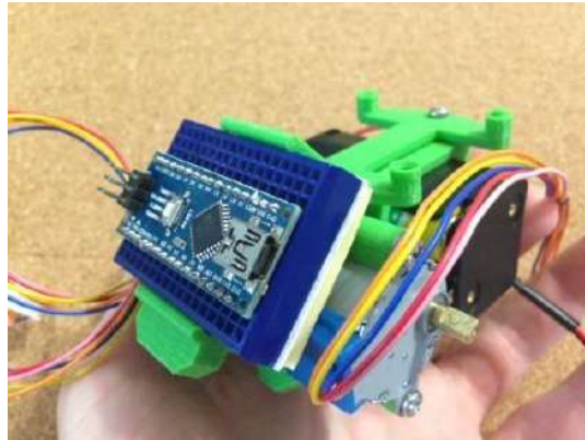
Figura 14. Montaje del protoboard.
