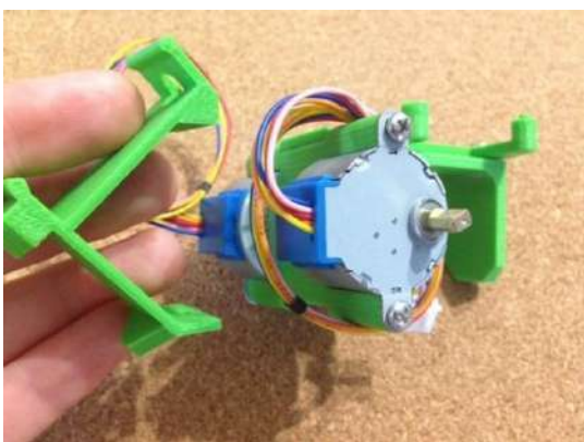
Figura 8. Soportes del motor
