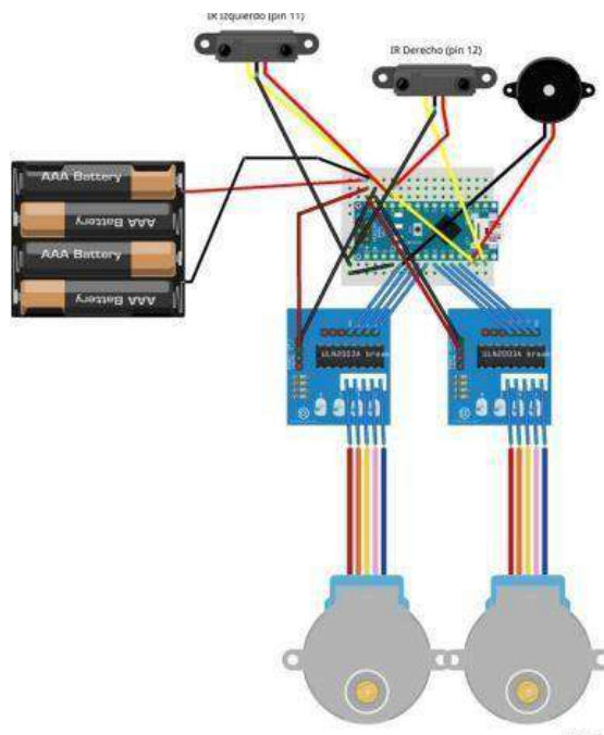
Figura 20. Conexiones generales.
