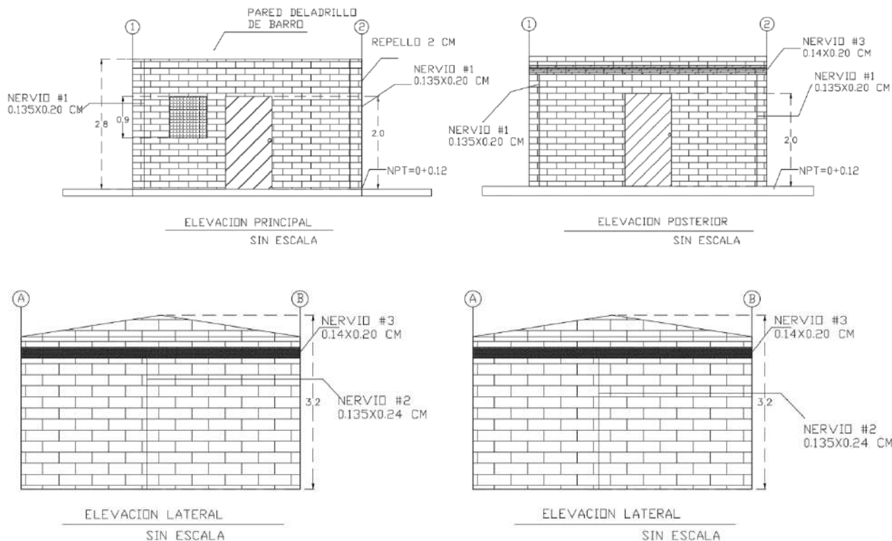
Plano 4. Detalle de Elevación.
