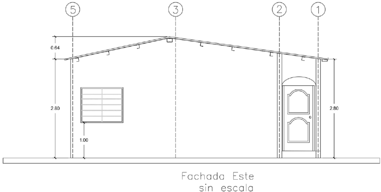
Plano 9. Fachada Este Fuente. Elaboración de HPH ES.
