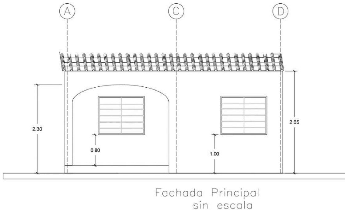
Plano 10. Plano de modulación. Fuente. Elaboración de HPH ES.
