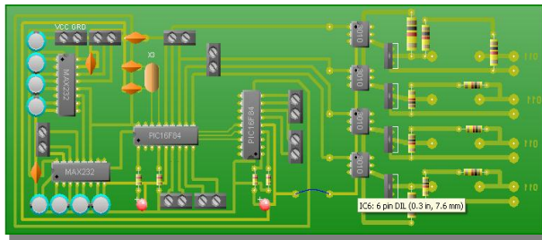
Figura ¡Error! No hay texto con el estilo especificado en el documento.-2. Circuito controlador desarrollado en el proyecto de investigación 2006.
