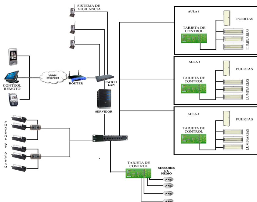
Figura ¡Error! No hay texto con el estilo especificado en el documento.-1. Esquema general del sistema
