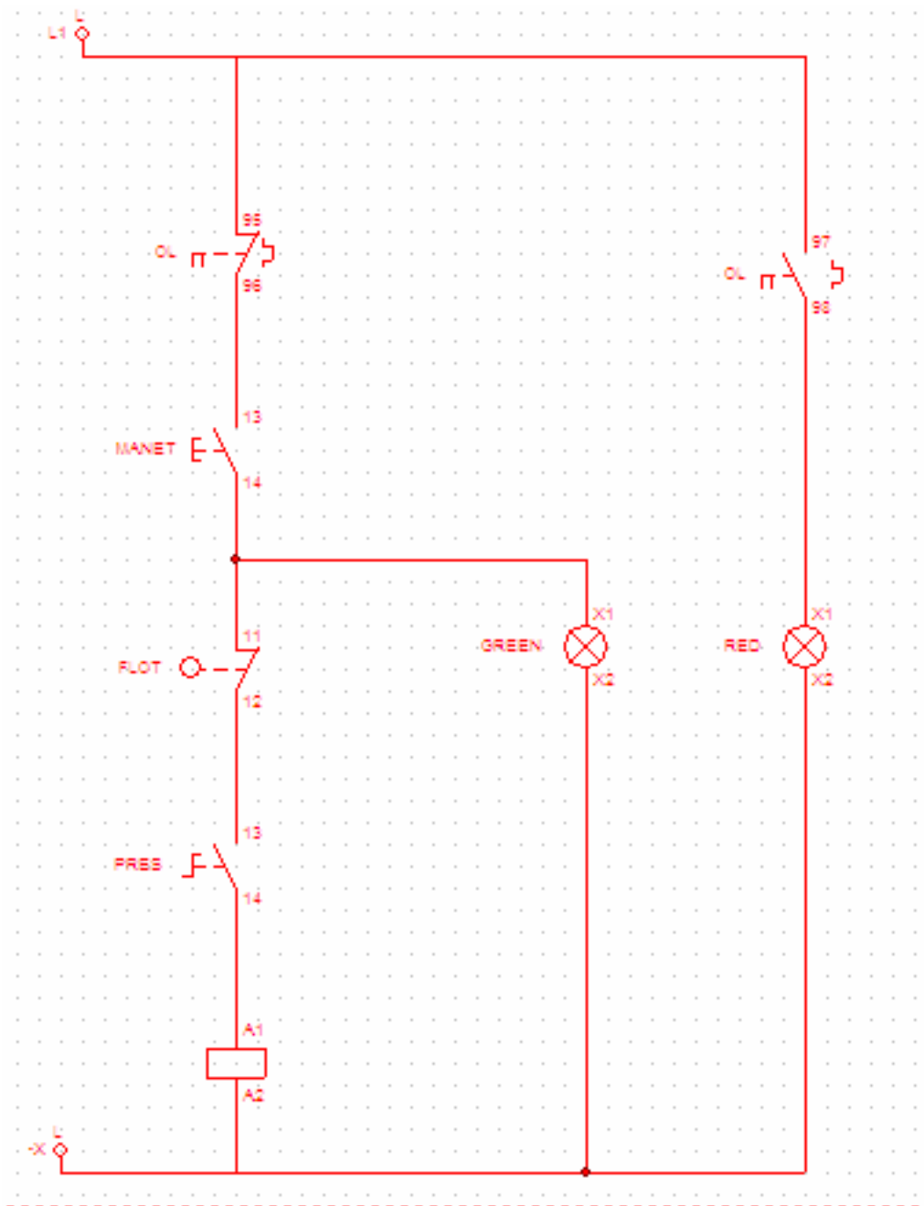
Figura ¡Error! No hay texto con el estilo especificado en el documento.-5. Diagrama de conexión del sistema de control automático
