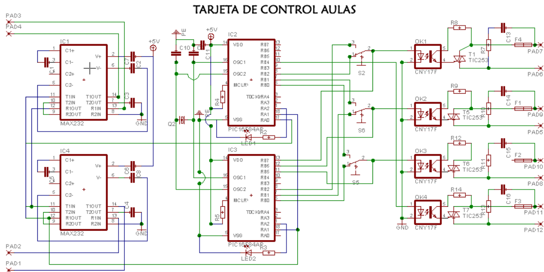
Figura ¡Error! No hay texto con el estilo especificado en el documento.-4. Tarjeta de control de las aulas
